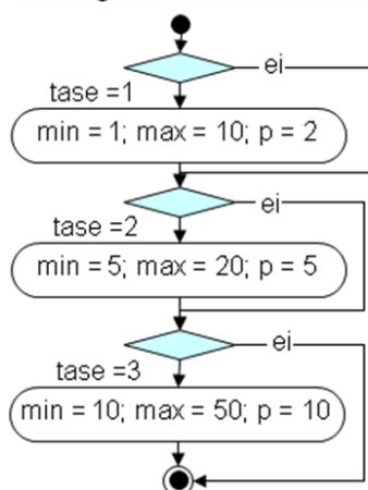
Tegevusskeem - UML
